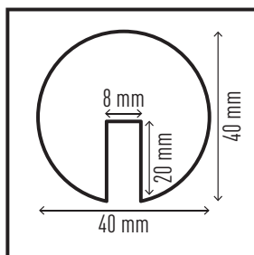
Profil ochronny do krawędzi E8R #1126-130
