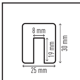
Profil ochronny do krawędzi E8 #1127-130
