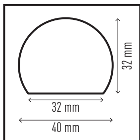
Profil ochronny do powierzchni S32R #1109-130
