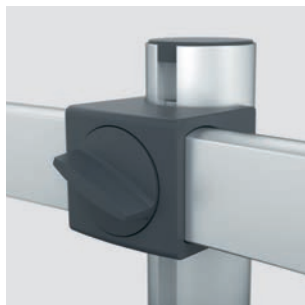
Ramię utrzymujące monitor o regulowanej wysokości od 50 do 340 mm, regulacja poprzez pokrętko
